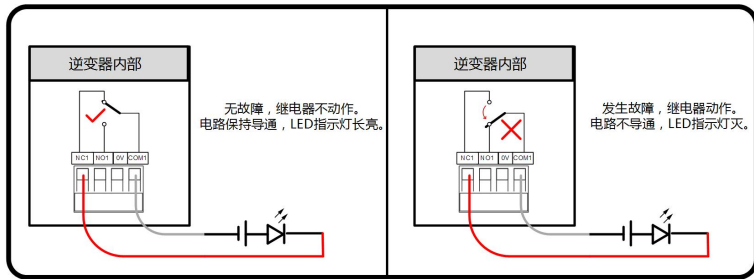
图 5-5 设置为常闭触点
