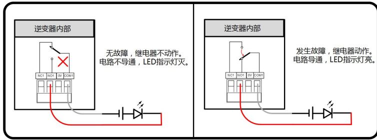
图 5-4 设置为常开触点
