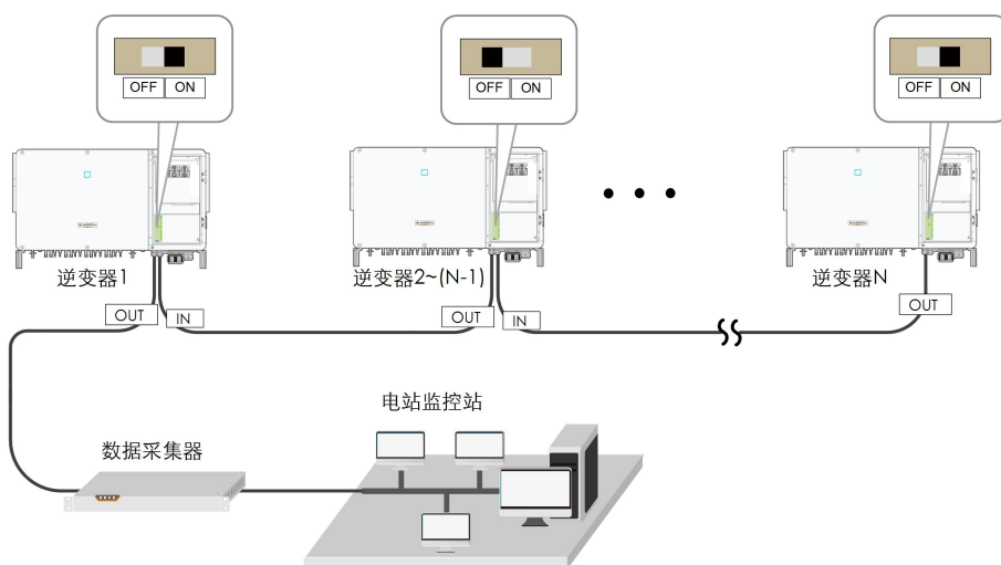
图 5-3 拨码开关配置 ( N \geq 15 )
