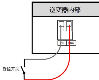
图 5-6 本地停止干接点典型应用
