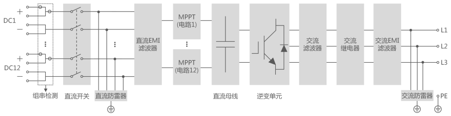
图 2-5 电路结构框图
