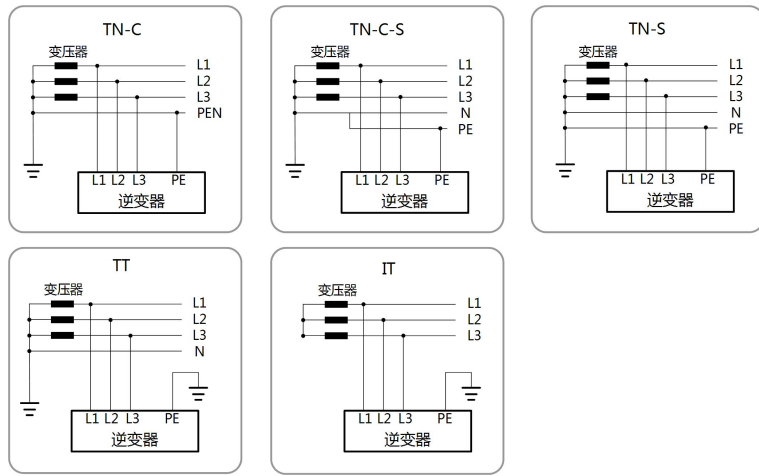
图 2-2 电网类型
