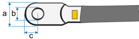
图 5-2 端子尺寸
