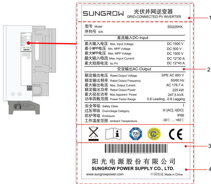
图 3-1 铭牌
