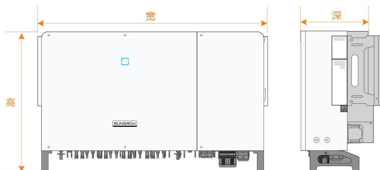
图 2-3 尺寸
